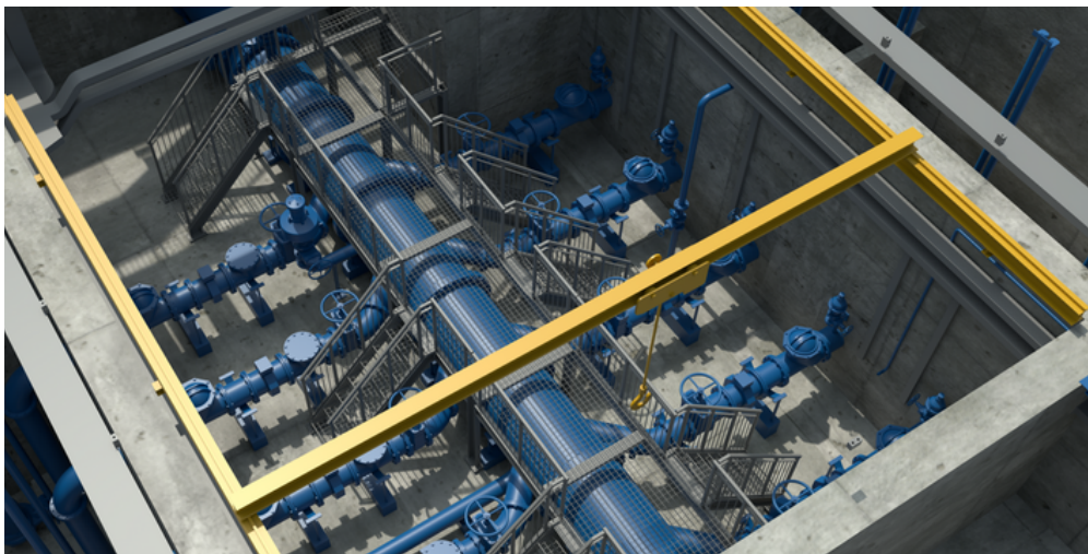
Immagine di modello informativo BIM di impianti idraulici ed elettrici, strutture in c.a. e di carpenteria metallica.
